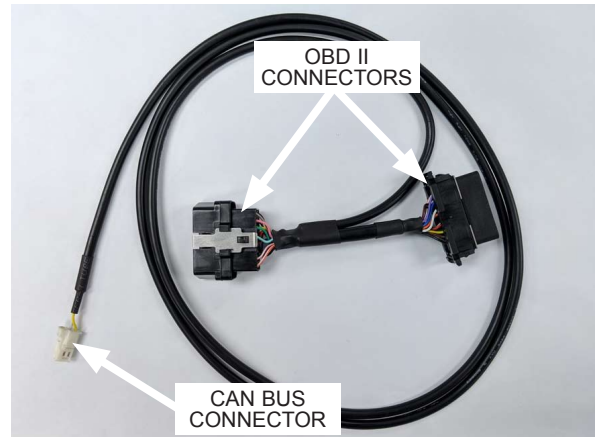
Fig. 11-a: Calibrator cable
