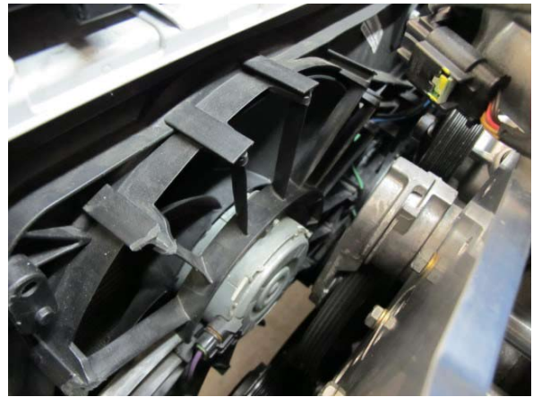
Fig. 2-n: Remove radiator fan assembly
