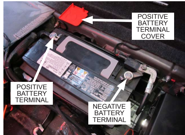
Fig. 1-a: Unplug battery
